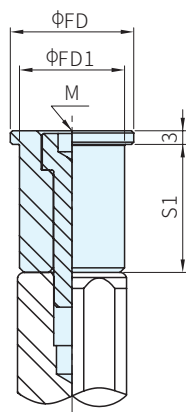
長固定蓋板
