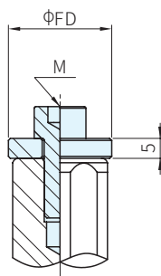
短固定蓋板
